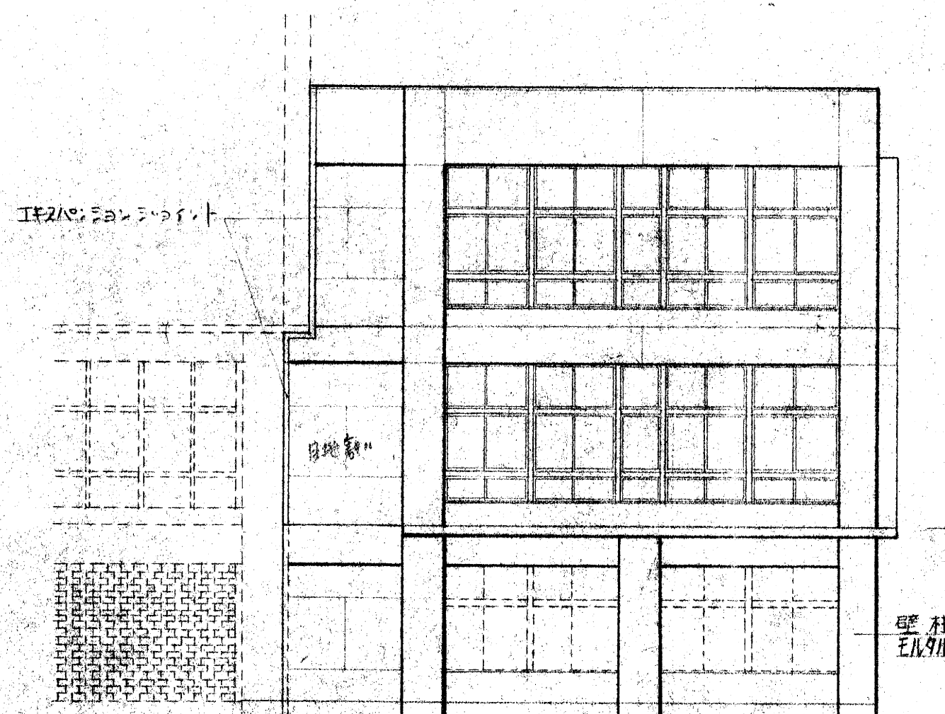
東側立面图 1:100
